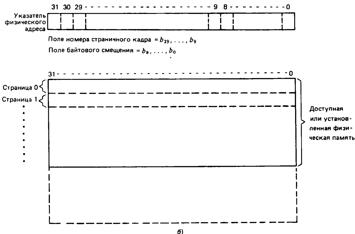
Рис. 10.7, б. Схема пространства физической памяти
