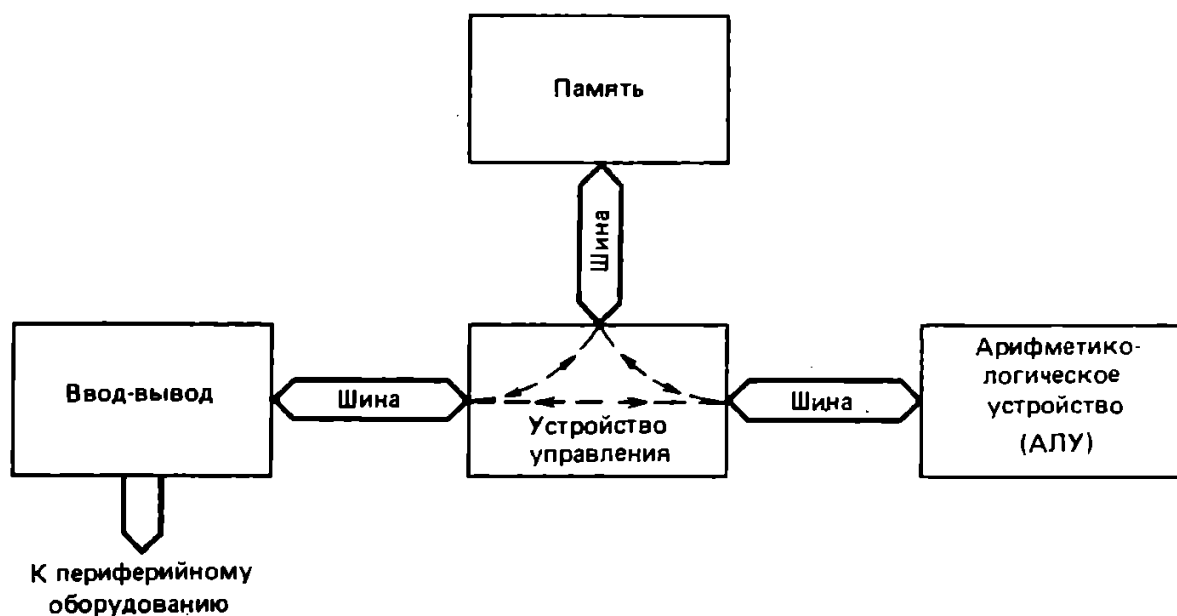
Рис. 1.1. Блок-схема базовой ЭВМ
