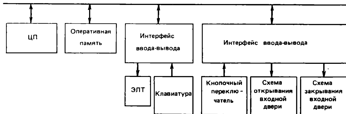
Рис. 7.9. Структура системы для контроллера защищенного входа в здание
