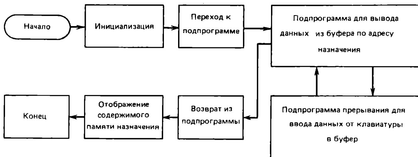
Рис. 8.8. Функциональная блок-схема системы
