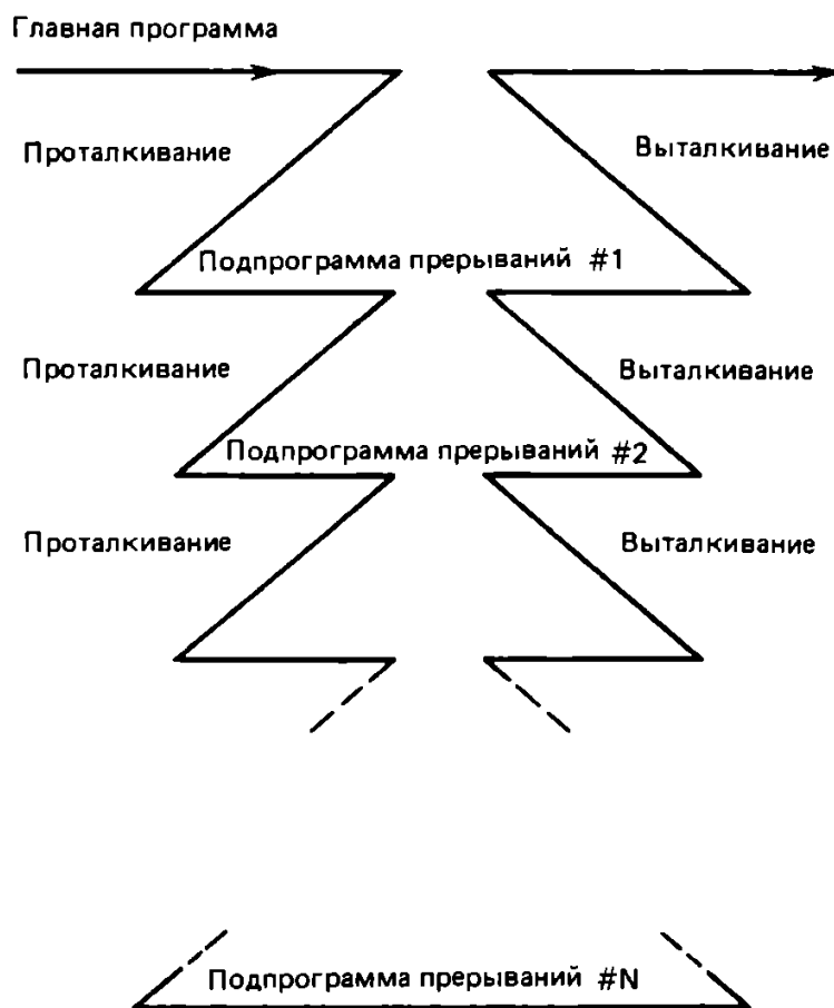
Рис. 8.20. Вложение прерываний
