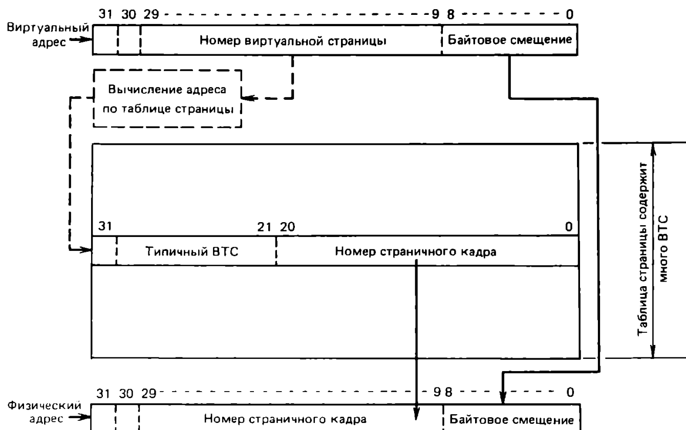
Рис. 10.9. Преобразования адреса
