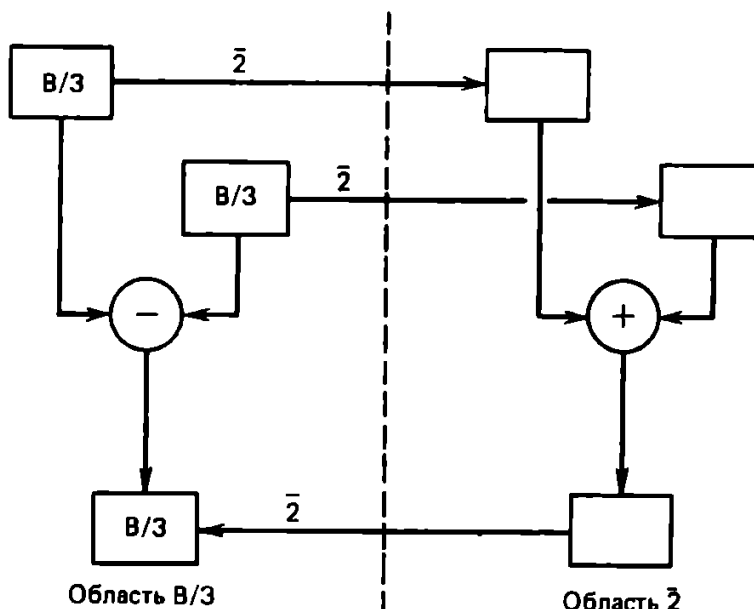
Рис. 3.2. Процесс выполнения вычитания путем сложения дополнений до двух
