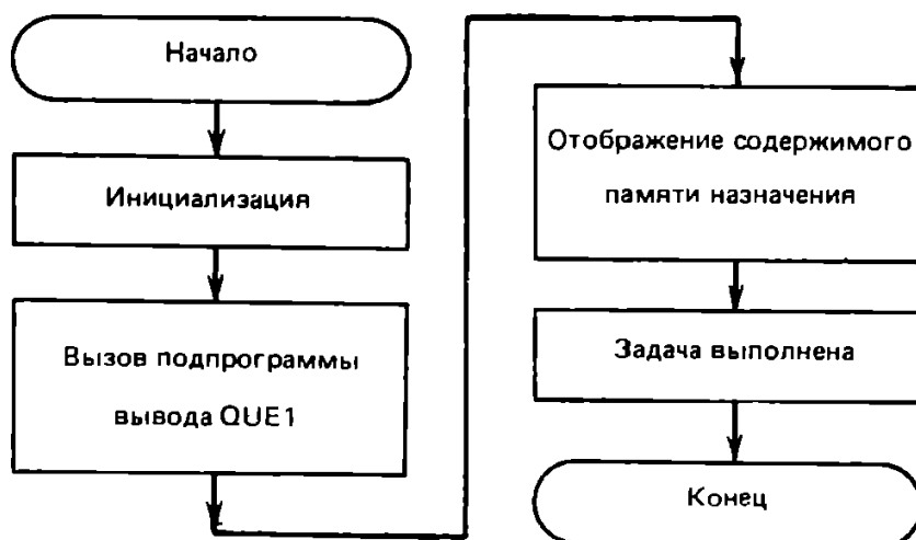
Рис. 8.9. Блок-схема главной программы QUE0
