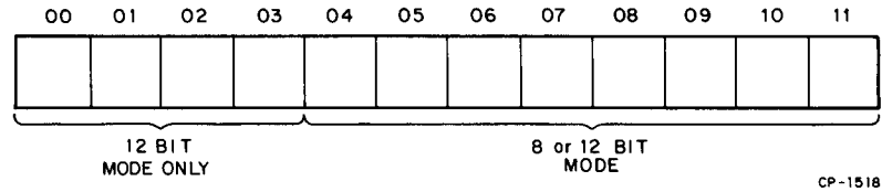
Figure 4-6 RXDB Format (RX8E)
