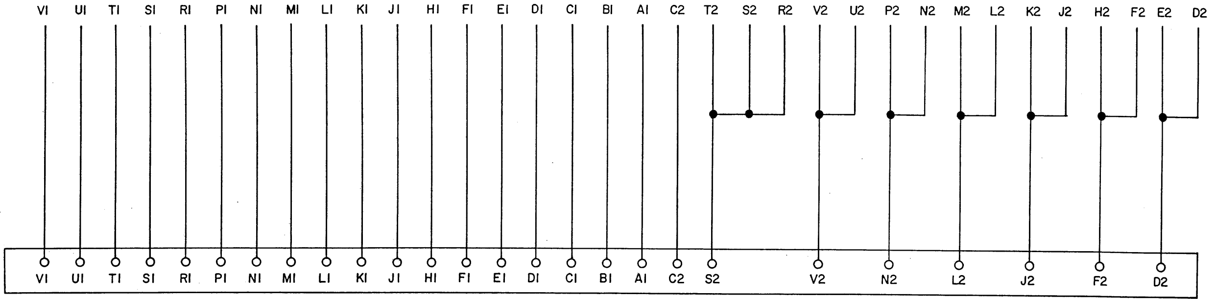
CONNECTOR 7900-0155-0
